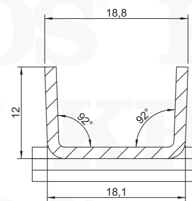
SEZIONE A-A
